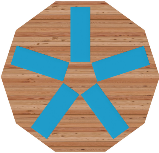
16ft Dome
