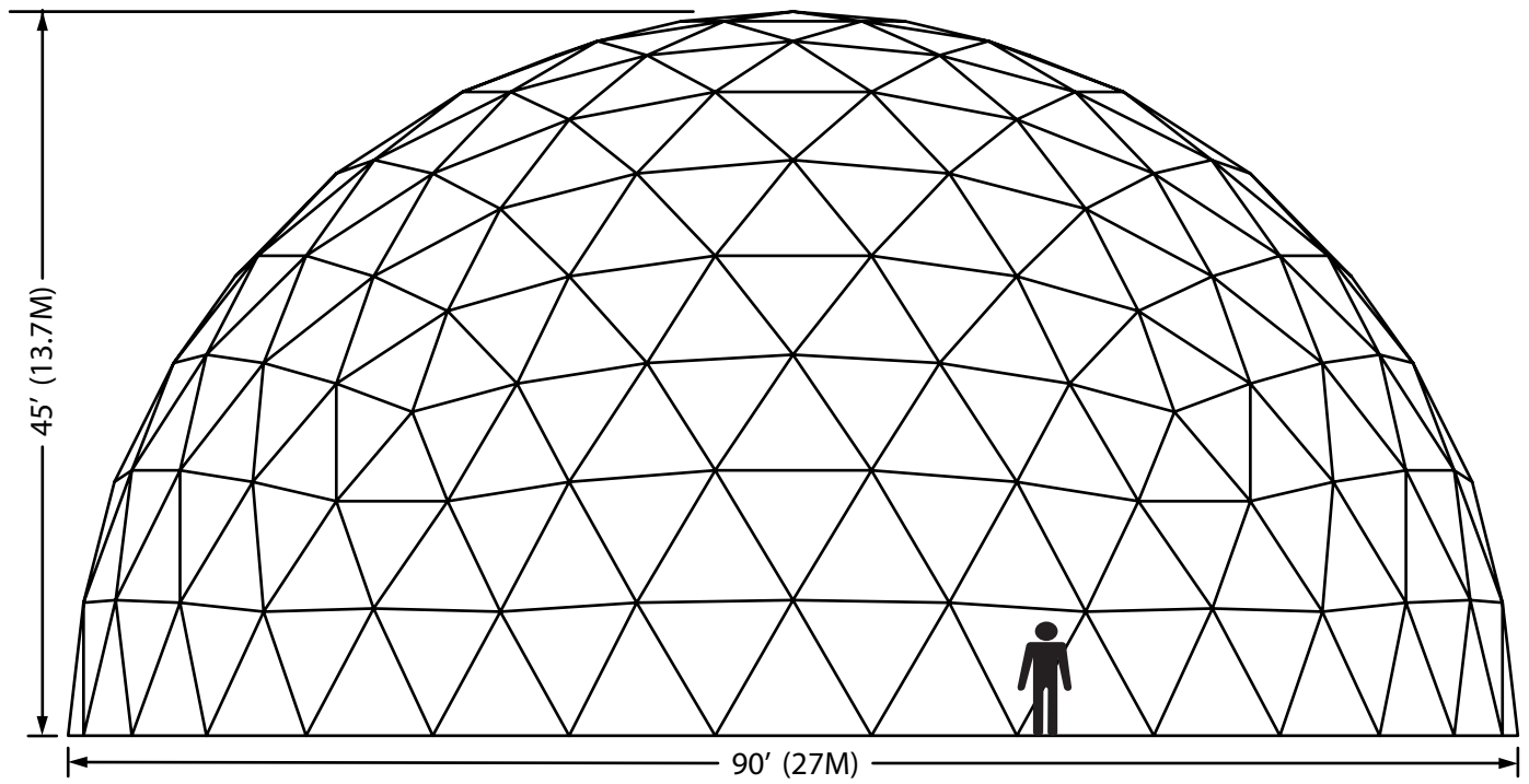
90' Dome Elevation
